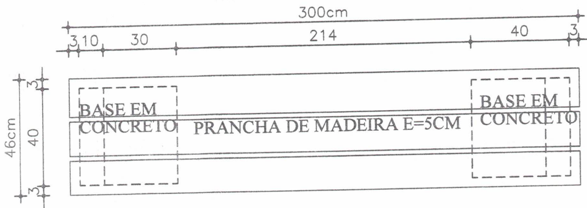
1 PLANTA BAIXA DO BANCO ESCALA: 1 / 30
