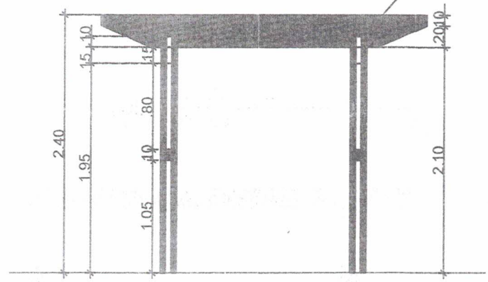
07 Vista Lateral - Pergolado ESC. 1/50
