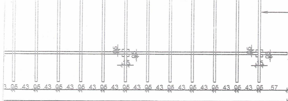
05 Planta Baixa - Pergolado ESC. 1/50
