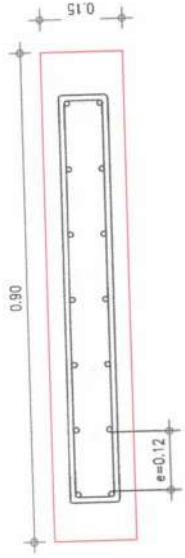
03 | SEÇÃO TRANSVERSAL DE TAMPALIAJE DE CONCRETO ESCALA 1:50C
