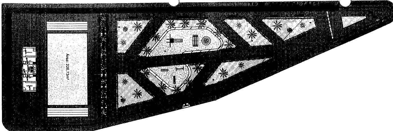
01 PLANTA PAGINAÇÃO DE PISOS - PRAÇA JOSÉ GERARDO ALVES
