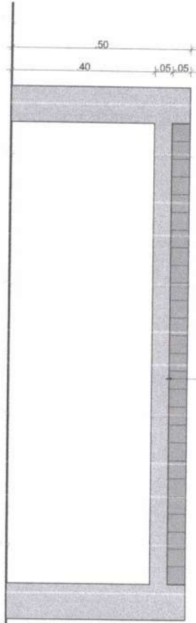
02 Vista Frontal - Banco 01 ESC. 1/10
